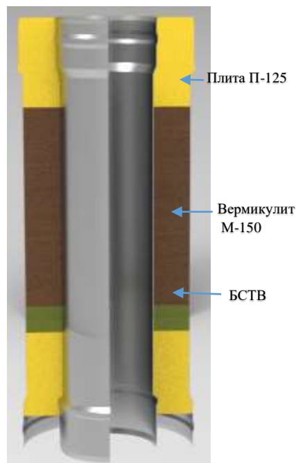
Рис.1. Первая группа элемента дымохода (сэндвич-труба)
