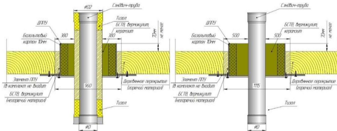
Рис.3 (А, Б). Устройство ППУ в перекрытии согласно СНиП 41-01-2003
