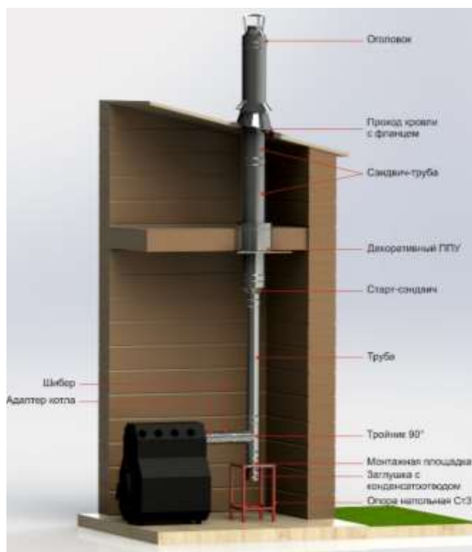
Рис.7 Двустенный вертикальный дымоход с проходом через потолочное перекрытие и кровлю, при горизонтальном выходном патрубке котла.
