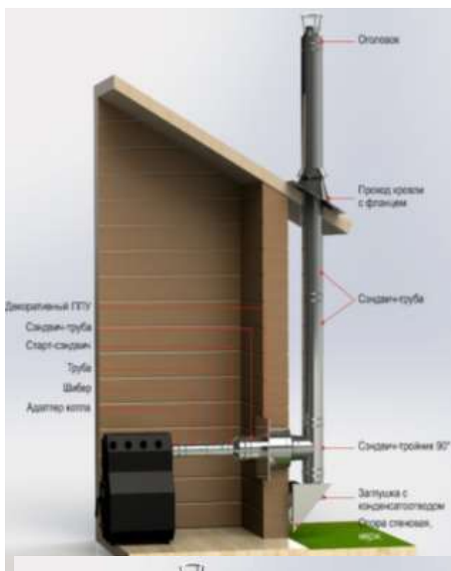
Рис.8 Двустенный вертикальный дымоход на внешней стороне стены с проходом через стену и кровлю при горизонтальном выходном патрубке котла.
